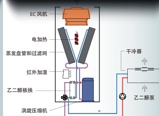
上送风-EC 风机
