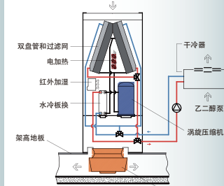
下送风-EC 风机
