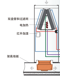
下送风-EC 风机
