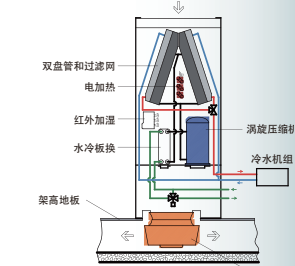
下送风-EC 风机
