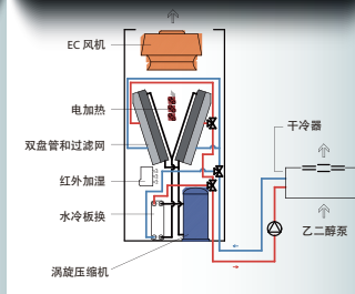
上送风-EC 风机
